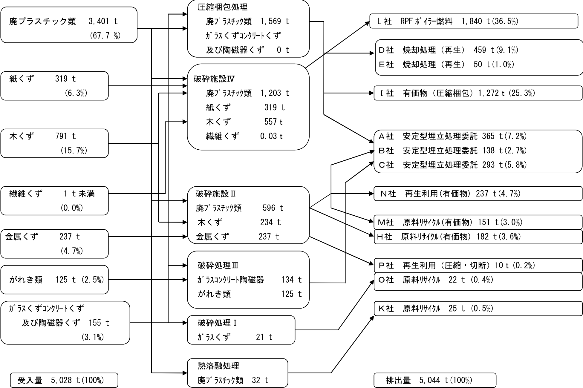
令和3年度 産業廃棄物受入・処分量フロー図
