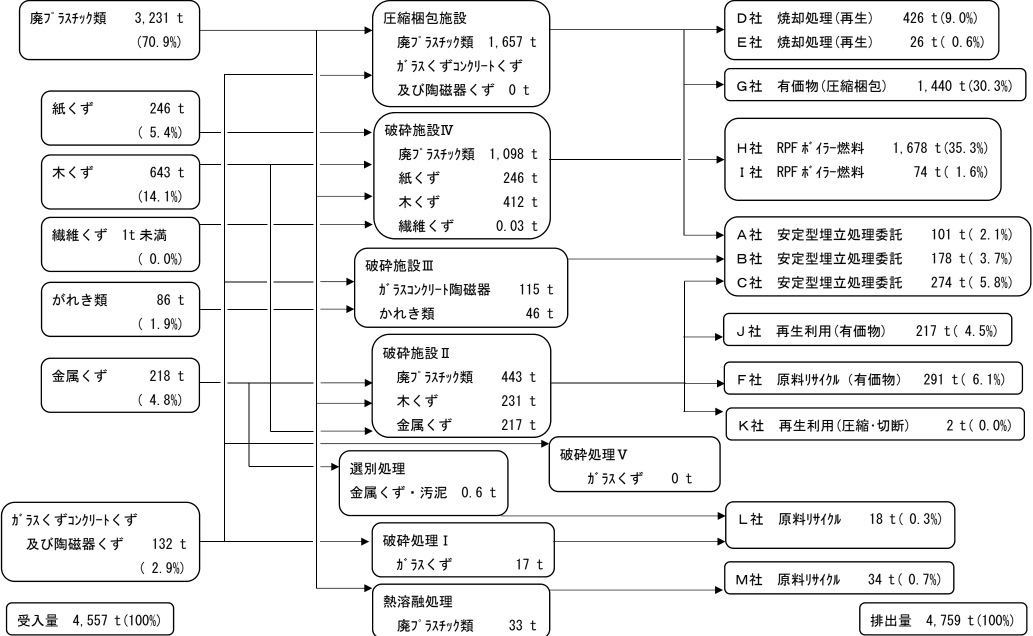
令和6年度 産業廃棄物受入・処理フロー図
